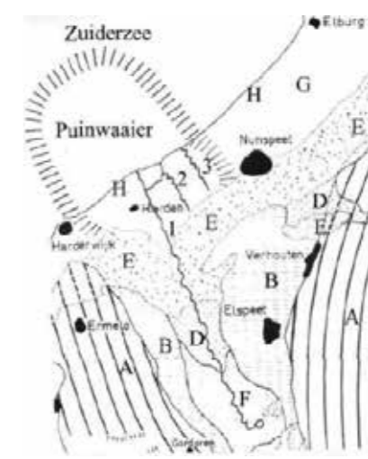
Uitsnede Geomorfische schets Veluwe; A=stuwwallen, B=smeltwaterafzettingen, D=dekzand, E=stuifzand, F=beekafzettingen, G=kustvlakte, H=strandwallen, 1=Hierdense Beek, 2=Killenbeek, 3=Nodbeek
