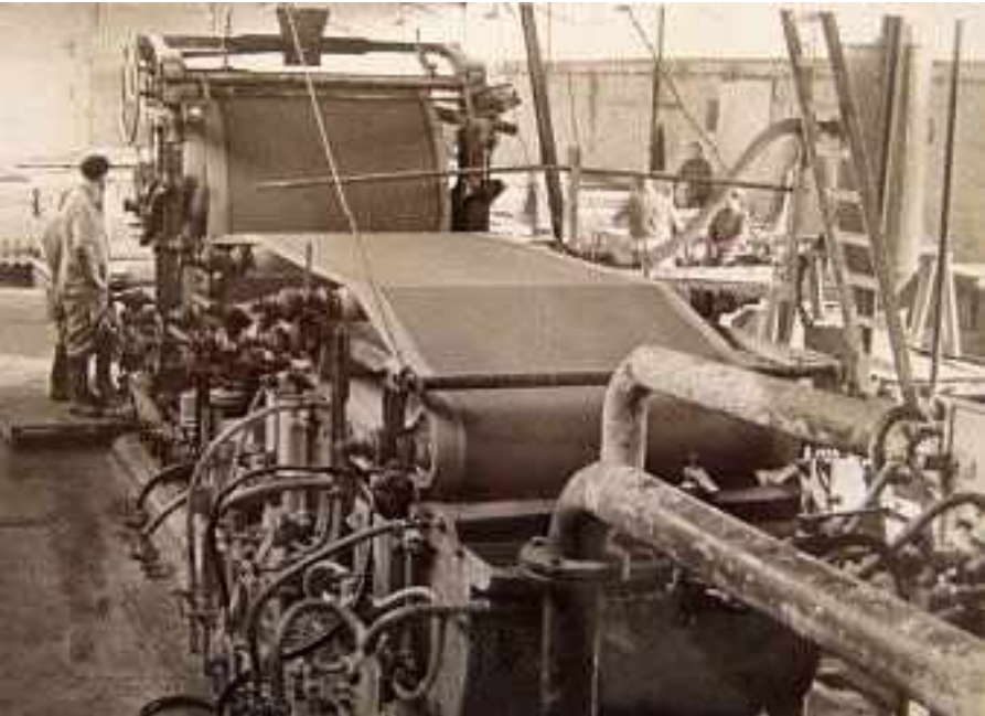
Een buizenmachine
