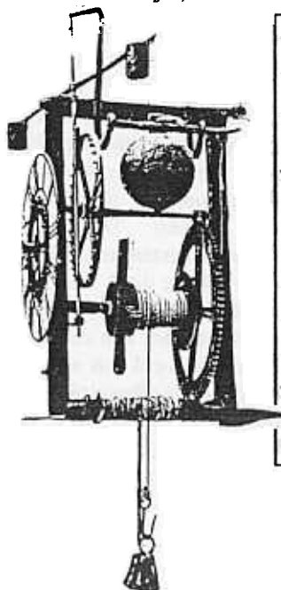
Een Gotisch torenwachtersuurwerk ±1380. In die tijd nog gemaakt door smeden i.p.v. klokkenmakers. Er is geen slinger. Er is een 'waag' als gangregeelaar.
