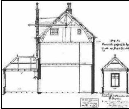
Kapconstructie 1903, tekening en uitvoering
